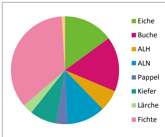
Baumartenanteile
